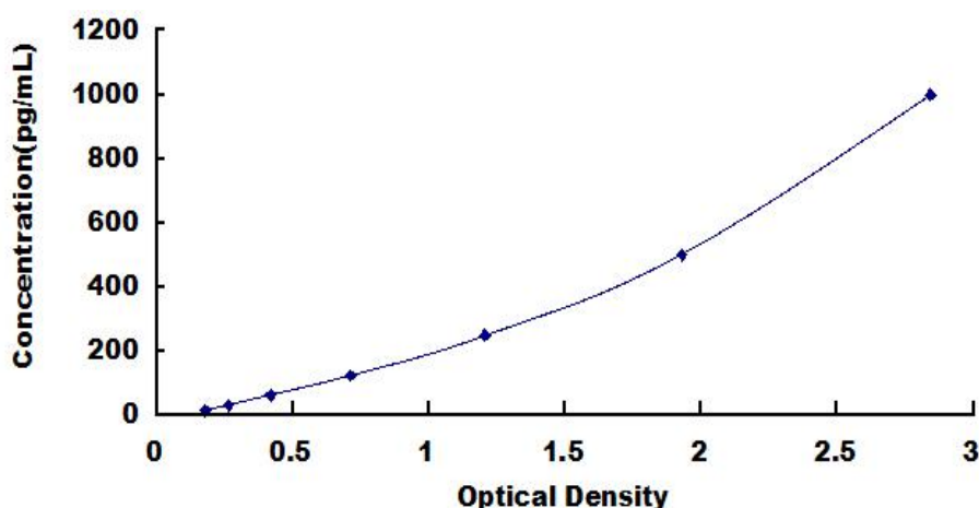
Typical Standard Curve for ANG ELISA.
